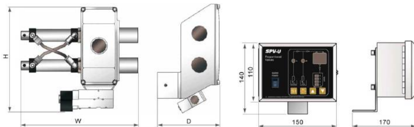
Корпус клапана
